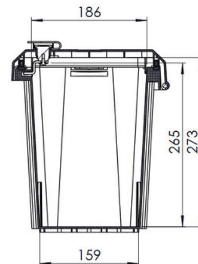
SEZIONE C-C
