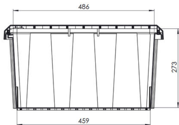
SEZIONE D-D
